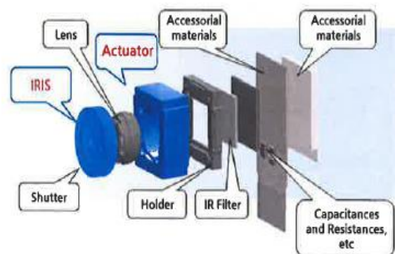
그림3. 카메라모듈 기본 구조
