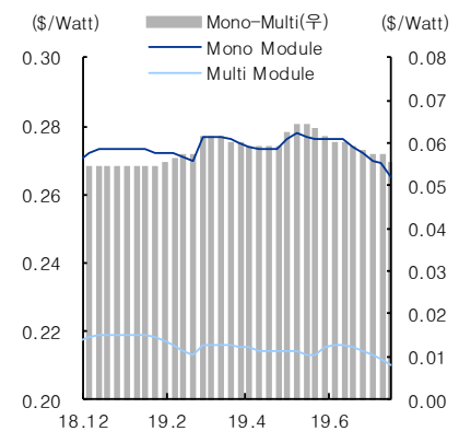
그림 27. 모듈 – Mono, Multi
