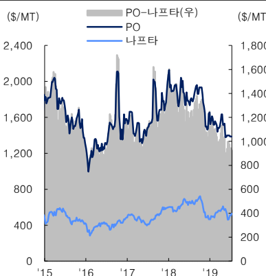
그림 17. PO-납사 스프레드
