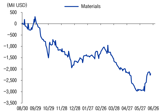
그림21 Materials Sector
