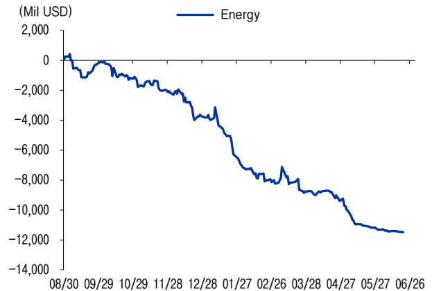
그림15 Energy Sector
