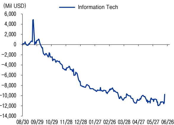
그림20 IT Sector
