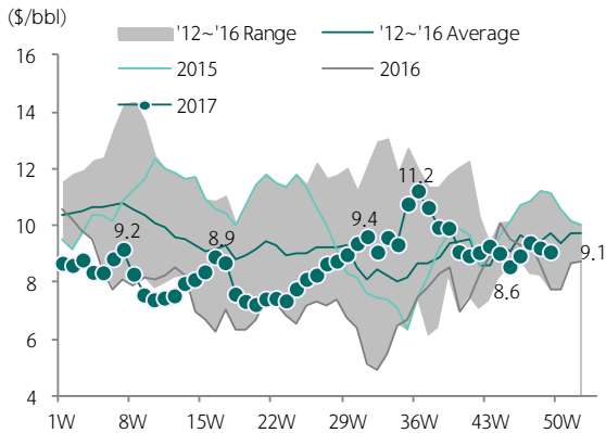
그림 27. 정제마진 추이
